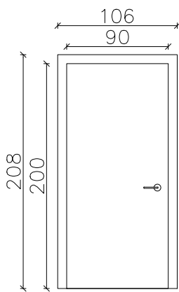
DRZWI DO POKOJU -NALEŻY DOSTOSOWAĆ MODEL DRZWI DO SZEROKOŚCI OTWORU DRZWIOWEGO -OPASKA 8cm
