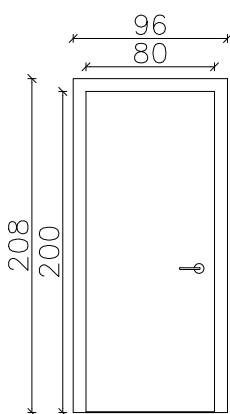
DRZWI DO MAŁEJ ŁAZIENKI -Z PODCIĘCIEM WENTYLACYJNYM NA CAŁĘJ DŁUGOŚCI -NALEŻY DOSTOSOWAĆ MODEL DRZWI DO SZEROKOŚCI OTWORU DRZWIOWEGO -OPASKA 8cm
