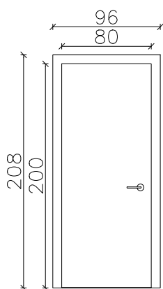
DRZWI DO DUŻEJ ŁAZIENKI -Z PODCIĘCIEM WENTYLACYJNYM NA CAŁĘJ DŁUGOŚCI -NALEŻY DOSTOSOWAĆ MODEL DRZWI DO SZEROKOŚCI OTWORU DRZWIOWEGO -OPASKA 8cm
